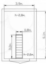
План гаража.
